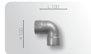
Curva 90° in alluminio pressofuso per il collegamento tra ponte-tubi.
