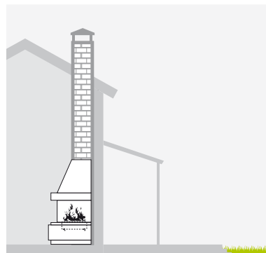
inserto braciere, installazione interna gas fire logs insert, indoor installation
